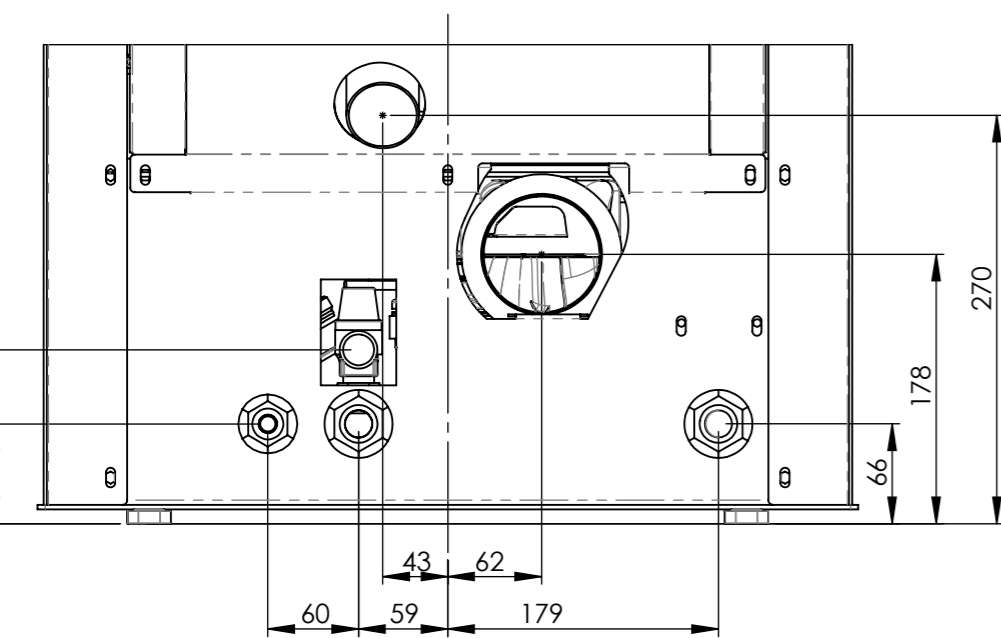
DETTAGLIO A SCALA 1 : 5
