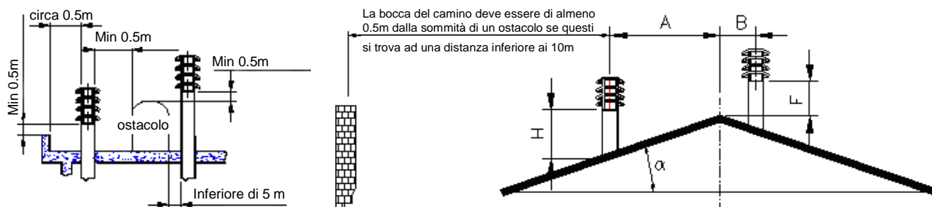
Fig. 2 Distances et positionnement des chapeaux
