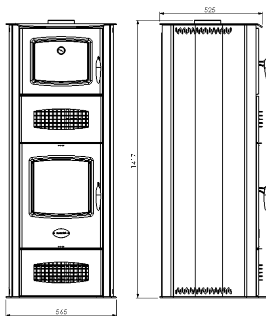
Fig 1 b Encombrement poêle Bea Forno
