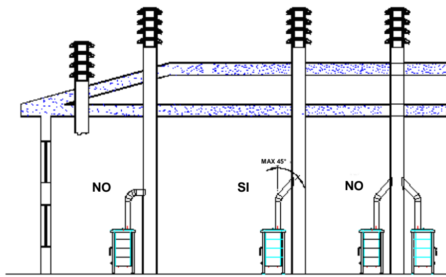
Fig. 3 Raccordement du poêle à la cheminée
