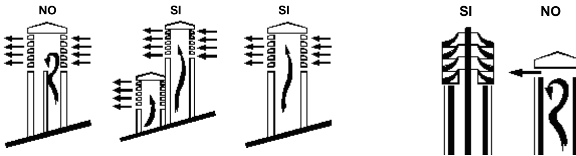
Fig 4 Réalisation de chapeaux de cheminée
