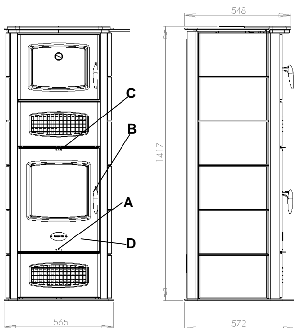
Fig 1 a Ingombri stufa Bea Forno (Maiolica)
